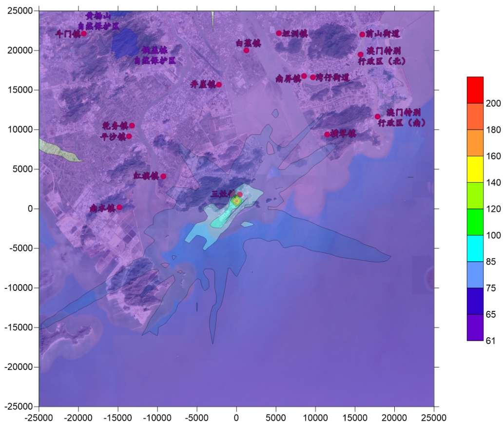
图 7-3-26 叠加现状后 PM 2.5 (包括一次和二次污染物) 保证率日均浓度等值线图 (µg/m 3 )
