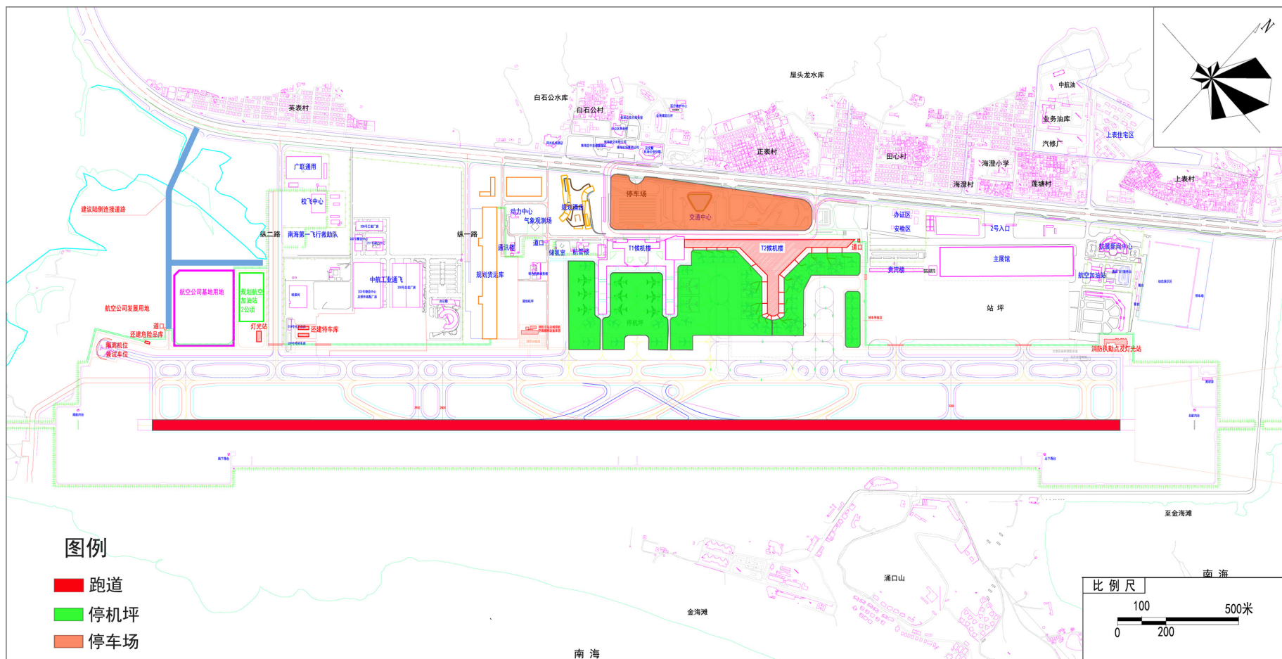
图 3-3-4 2027 年珠海机场环境空气污染源
