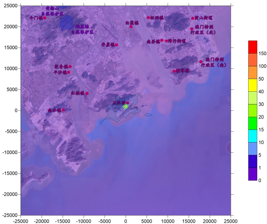
图 7-3-16 PM 10 日平均最大贡献浓度等值线图 (µg/m 3 )
