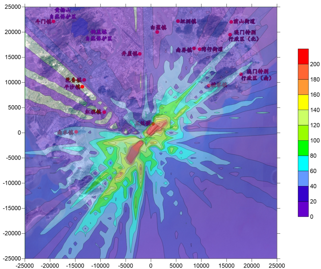
图 7-3-1 NO 2 小时最大贡献浓度等值线图 (µg/m 3 )
