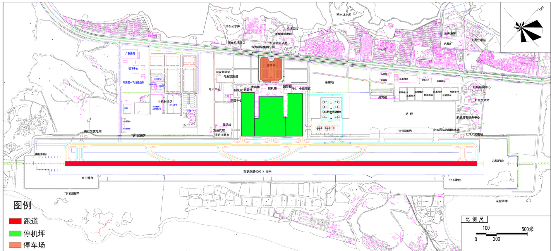
图 3-1-3 珠海机场现状环境空气污染源
