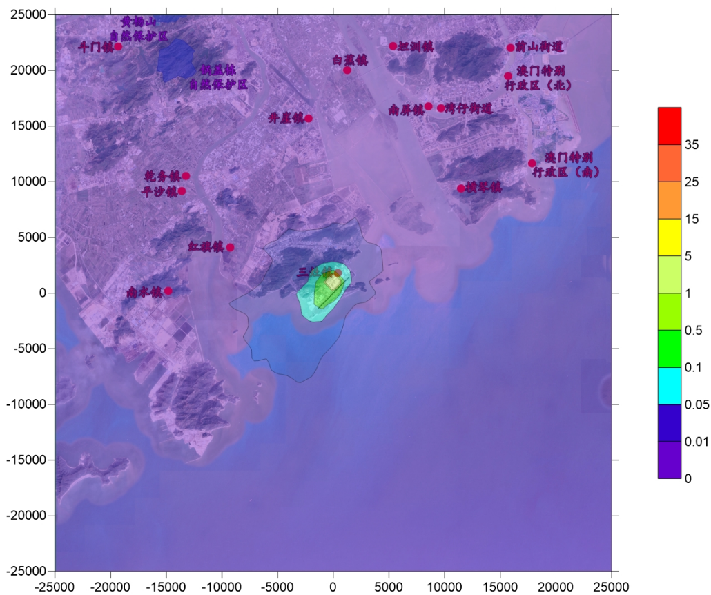
图 7-3-21 PM 2.5 (一次污染物) 年平均贡献浓度等值线图 (μg/m 3 )
