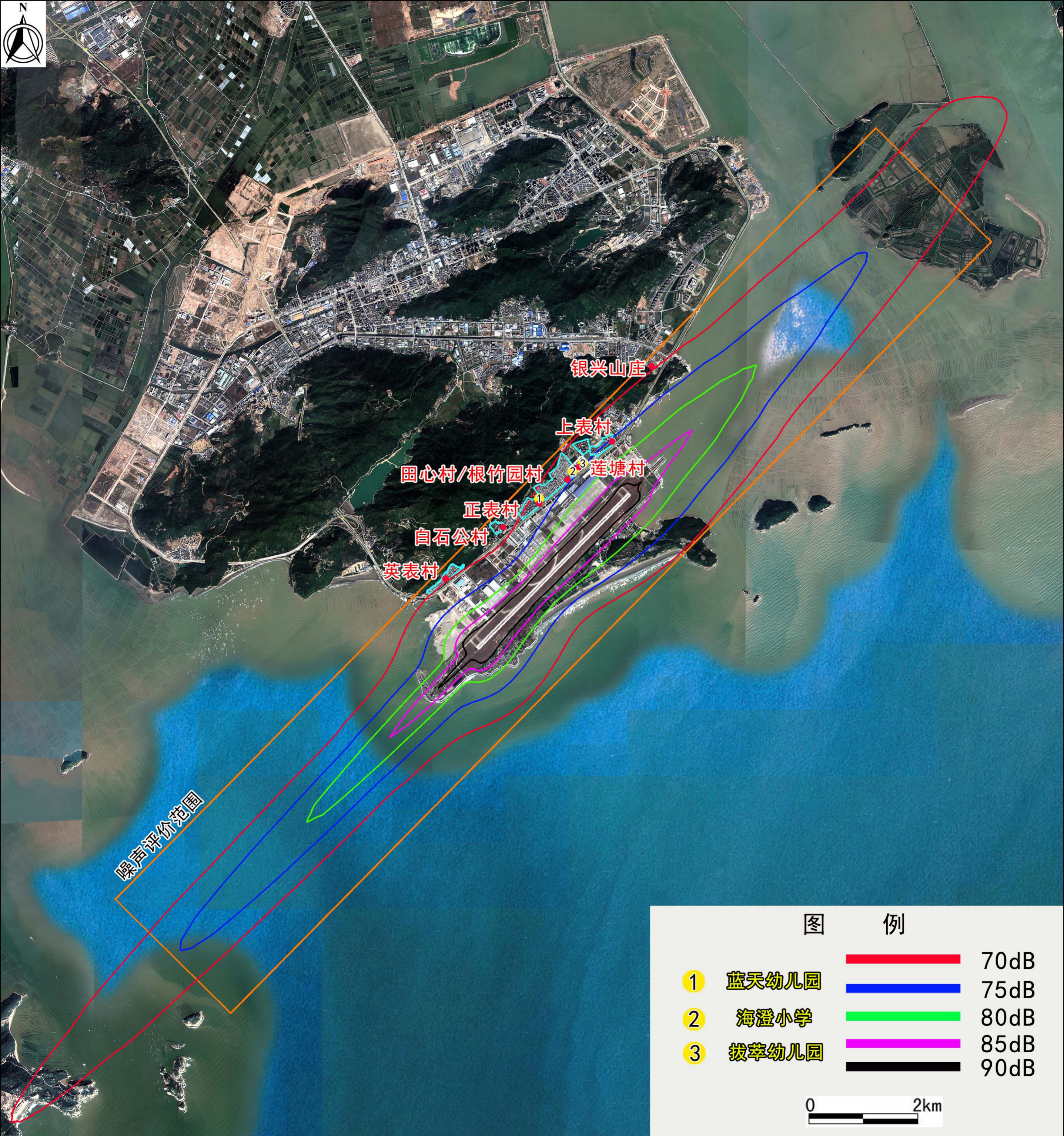
图6-2-10 珠海机场2027年飞机噪声等值线图
