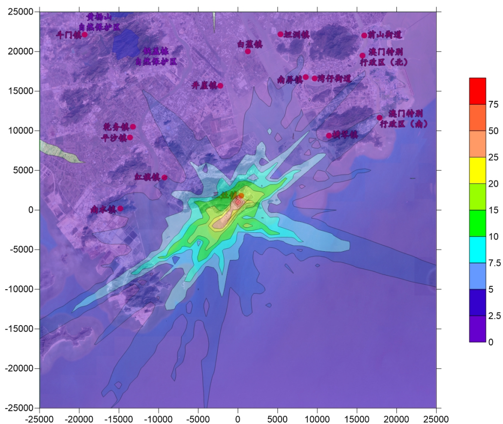
图 7-3-24 PM 2.5 (包括一次污染物和二次污染物) 日平均最大贡献浓度等值线图 (µg/m 3 )
