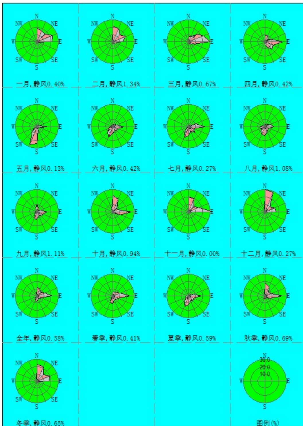
图 7-1-7 珠海机场 2018 年风频玫瑰图
