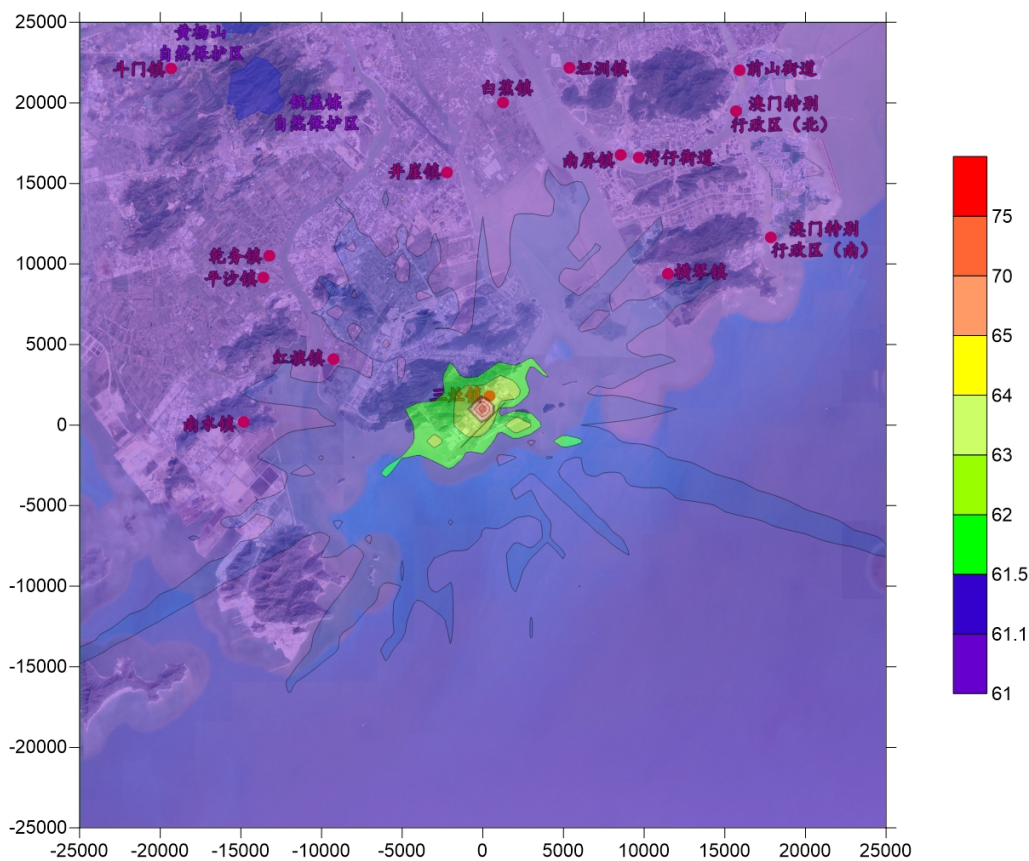
图 7-3-22 叠加现状浓度后 PM 2.5 (一次污染物) 保证率日平均质量浓度等值线图 ( \mu\text{g}/\text{m}^3 )
