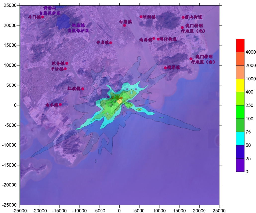
图 7-3-7 CO 日平均最大贡献浓度等值线图 (µg/m³)
