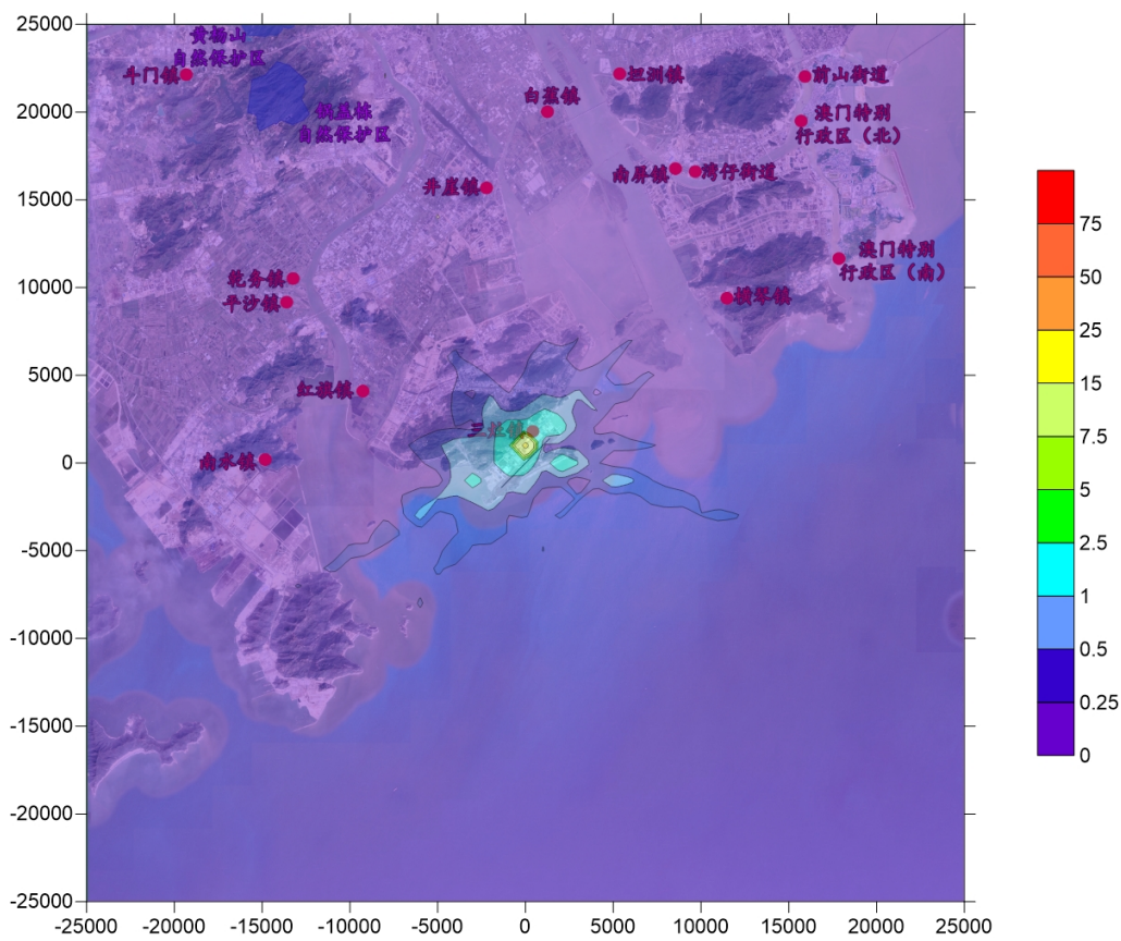
图 7-3-20 PM 2.5 (一次污染物) 日平均最大贡献浓度等值线图 (μg/m 3 )
