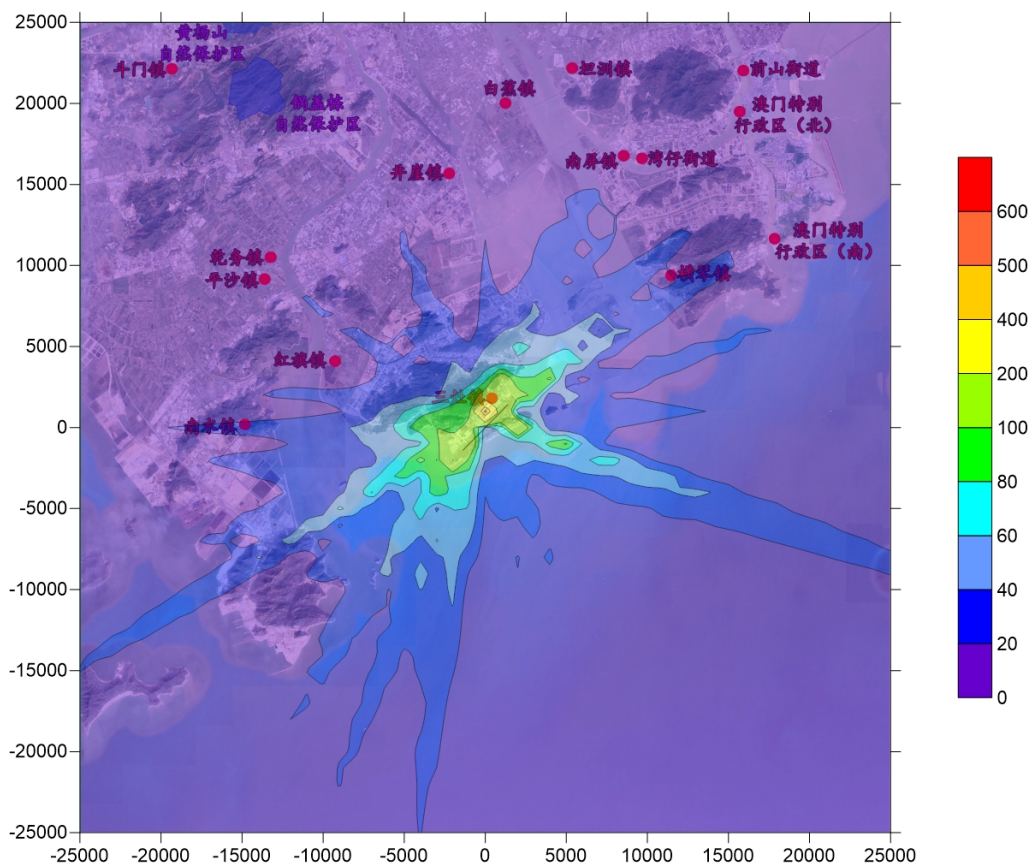
图 7-3-28 VOC 8 小时最大贡献浓度等值线图
