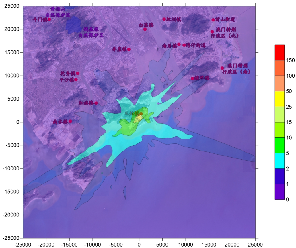
图 7-3-10 SO 2 日平均最大贡献浓度等值线图 (µg/m 3 )
