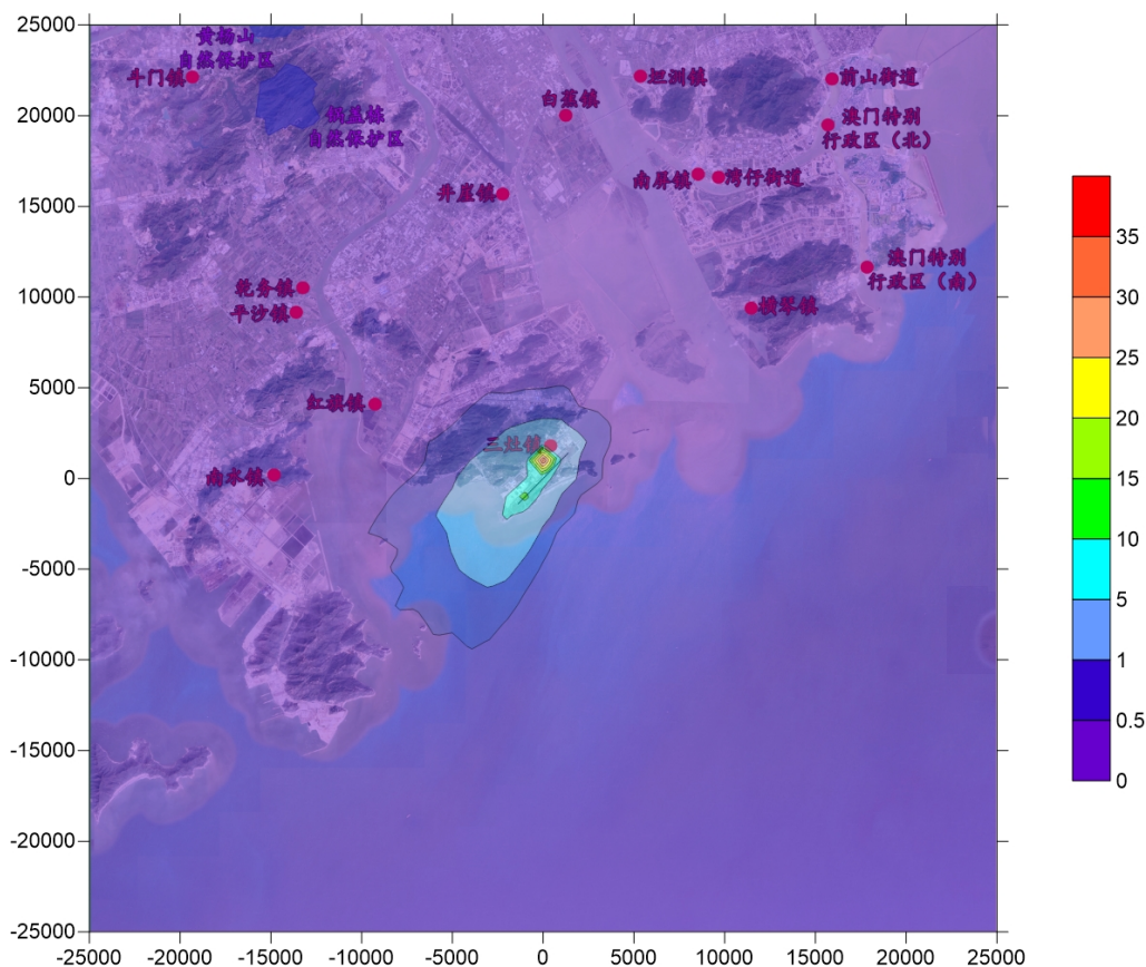
图 7-3-25 PM_{2.5} (包括一次污染物和二次污染物) 年平均贡献浓度等值线图 ( \mu\text{g}/\text{m}^3 )
