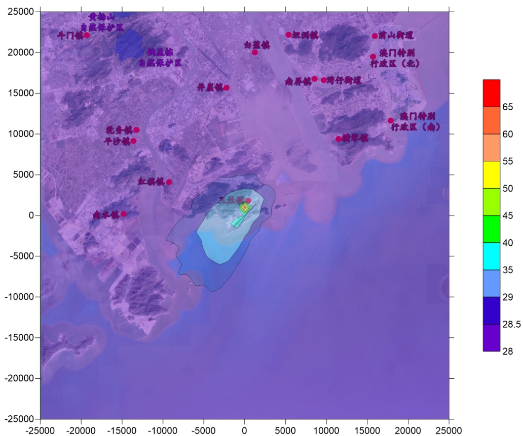
图 7-3-27 叠加现状浓度后 PM 2.5 (包括一次和二次污染物) 年平均浓度等值线图 (µg/m 3 )
