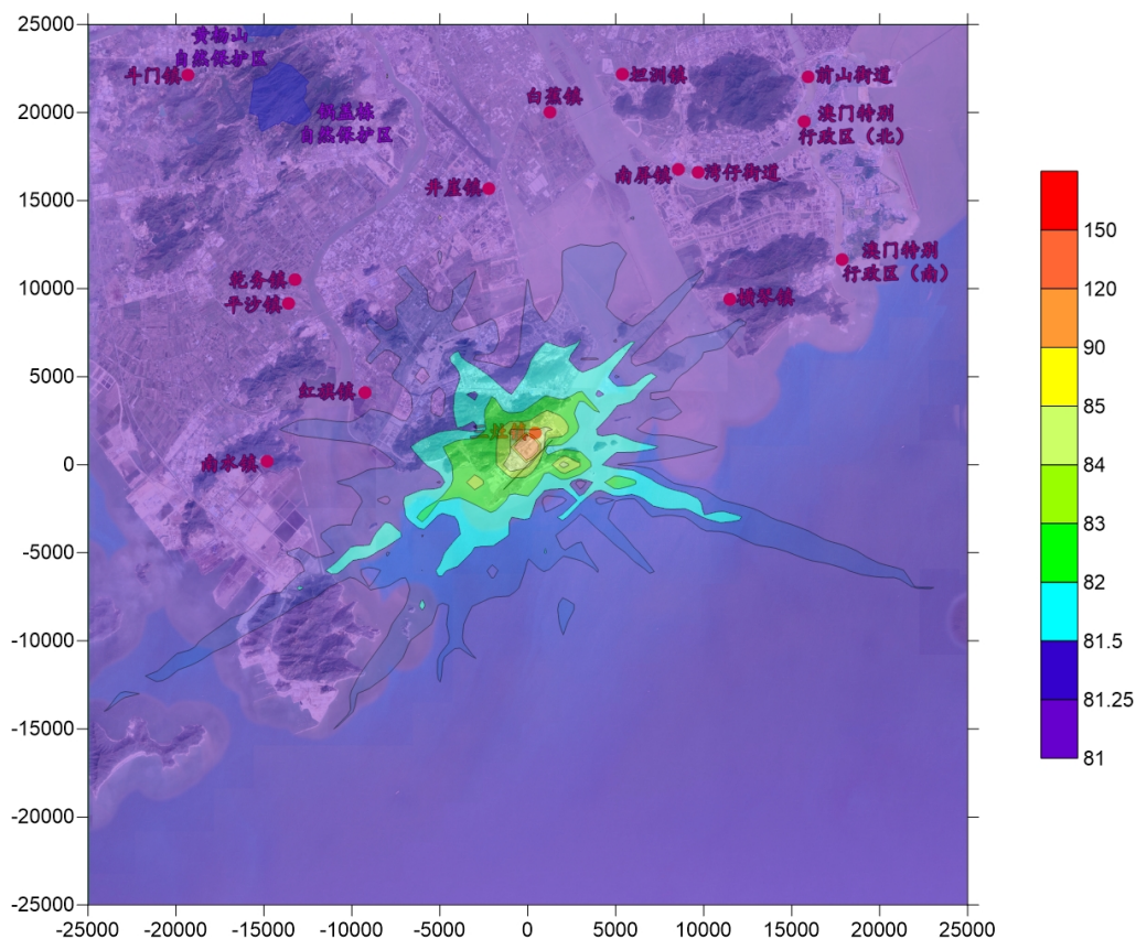
图 7-3-18 叠加现状浓度后 PM 10 保证率日平均质量浓度等值线图 (µg/m 3 )
