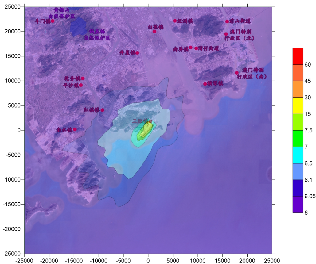
图 7-3-13 叠加现状浓度后 SO 2 年平均浓度等值线图 (µg/m 3 )
