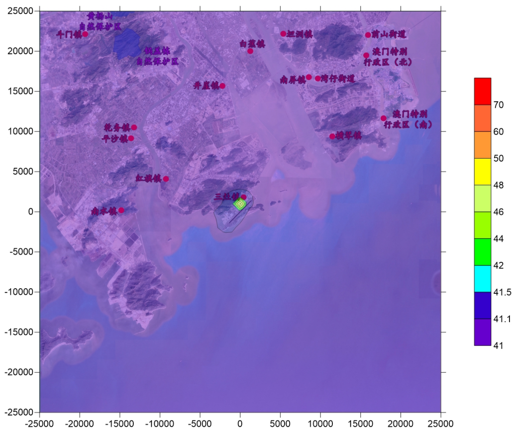
图 7-3-19 叠加现状浓度后 PM 10 年平均浓度等值线图 (µg/m 3 )
