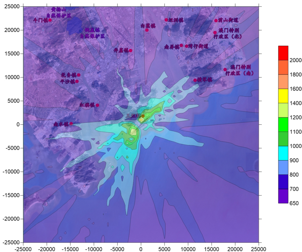
图 7-3-15 叠加现状浓度后 NMHC 小时质量浓度等值线图 ( \mu\text{g}/\text{m}^3 )
